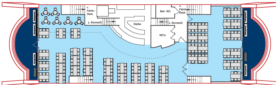
Restaurantdeck
